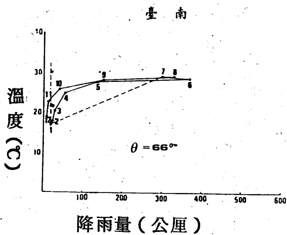
(圖十之b) Cwa 氣候
