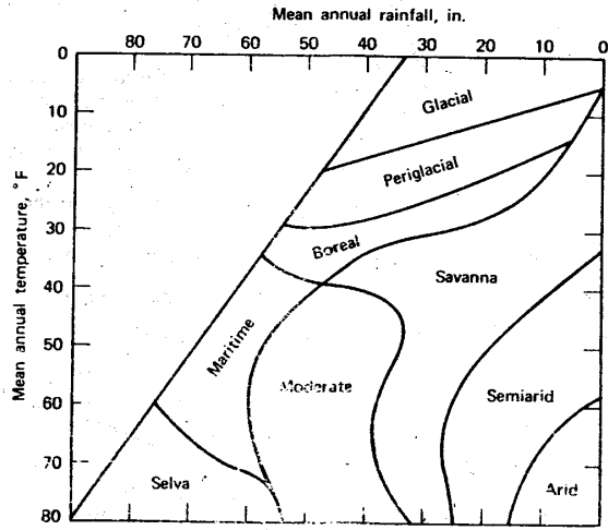
(圖四) 氣候地形圖 ( Peltier, 1950 )
