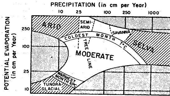
(圖五) 氣候地形圖 ( Tanner, 1961 )
