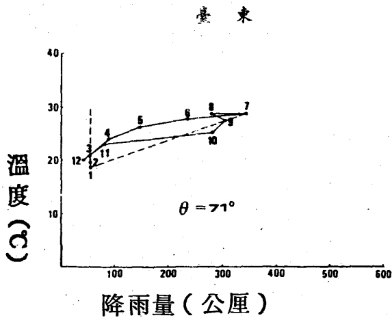
(圖十之 d) Am 氣候
