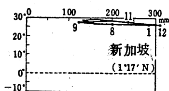
(a) Af Am
