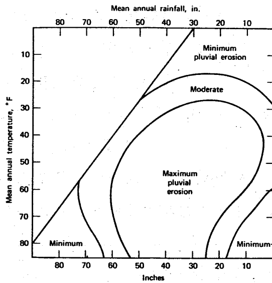
(圖三) 不同氣候下的降水侵蝕強度 ( Peltier, 1950 )
