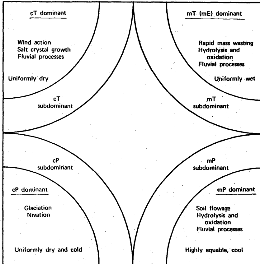
(圖七) 氣團與氣候地形關係圖 ( Oliver, 1972 )
